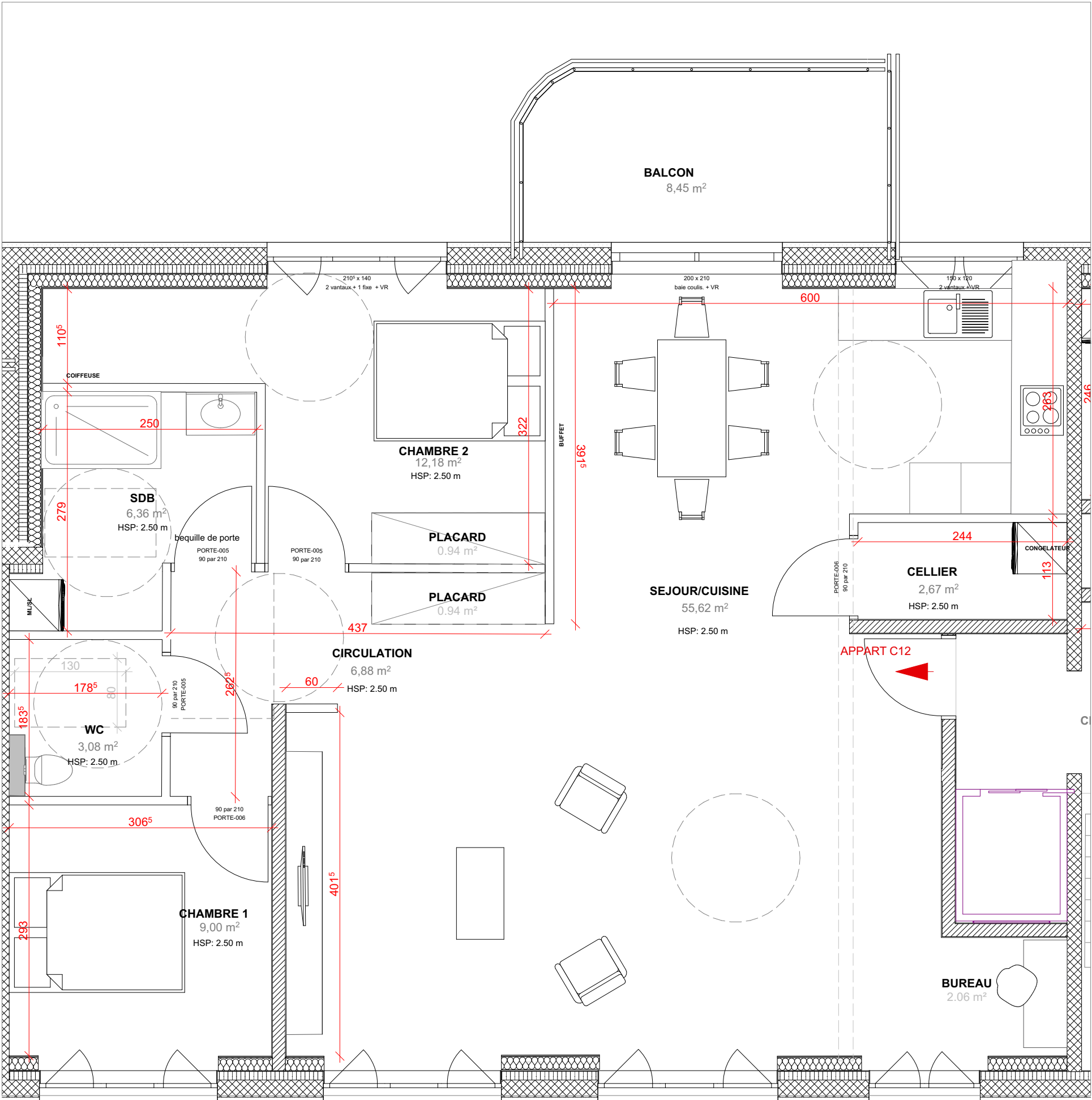
R+1 - 1/100e
