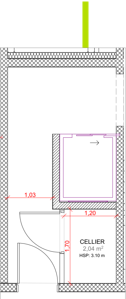
RDC - 1/50e
