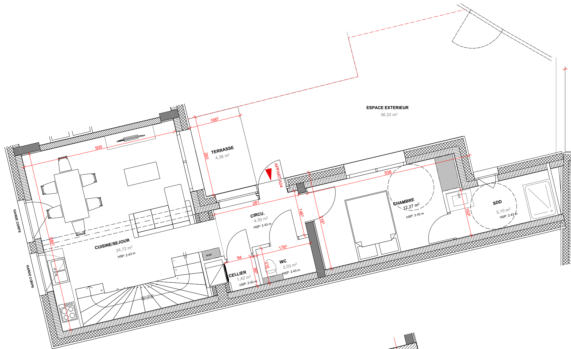
-- REZ-DE-CHAUSSEE --
