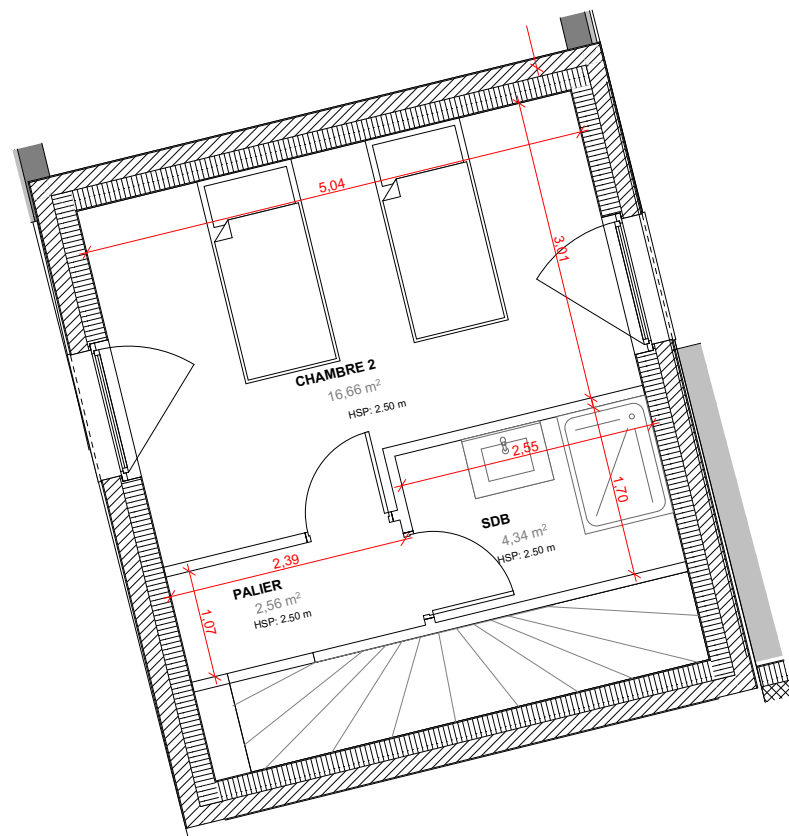
-- 1ER ETAGE --
